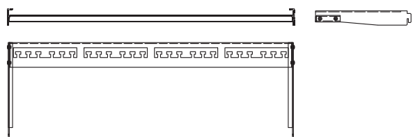
Nosač kablova za peč panel 19" - NKPP 24PR
